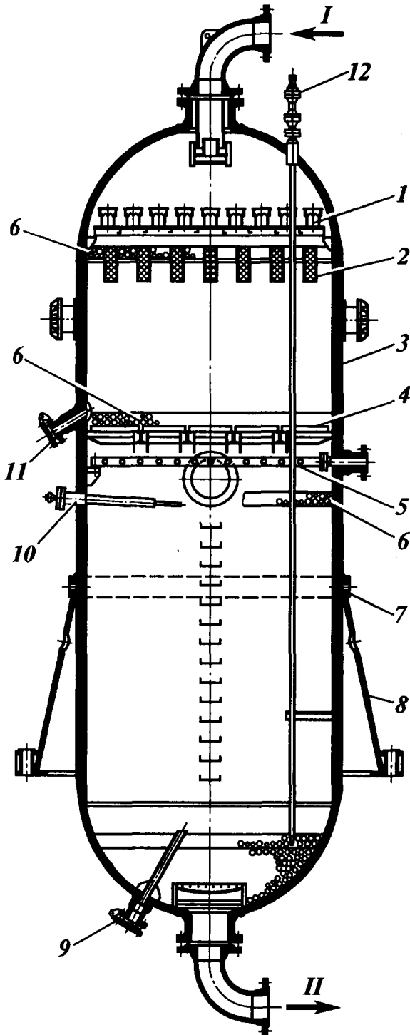
Рис. XXIV-2. Реактор гидроочистки дизельного топлива с аксиальным движением сырья: 1 — распределительная тарелка; 2 — фильтрующее устройство; 3 — корпус; 4 — решетка колосниковая; 5 — коллектор для ввода пара; 6 — фарфоровые шары; 7 — опорное кольцо; 8 — опора; 9, 11 — штуцер для выгрузки катализатора; 10, 12 — термометры. Поток: I — сырье; II — продукты реакции
